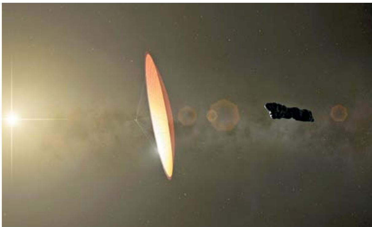
Représentation d' Oumuamua sous la forme d'une photovoile d'après Avi Loeb (à gauche), et sa représentation conventionnelle : un rocher allongé en forme de cigare (à droite).
